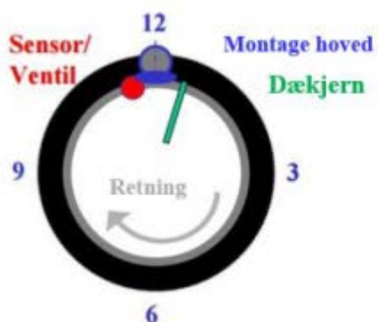
Fig. 1: Øverste kantråd
