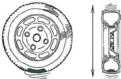
Fig. 1: Statisk ubalance.
